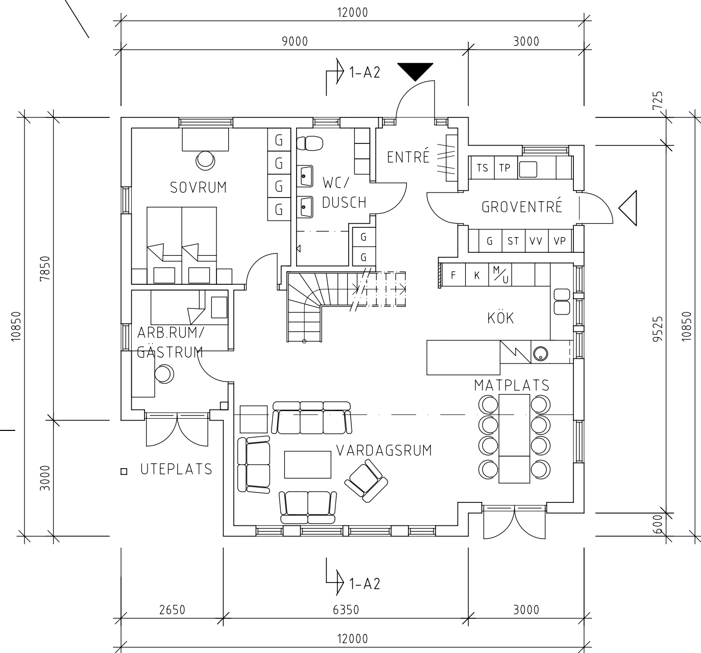
ENTRÉVÅNING
