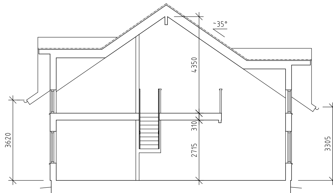
SEKTION 1-1
